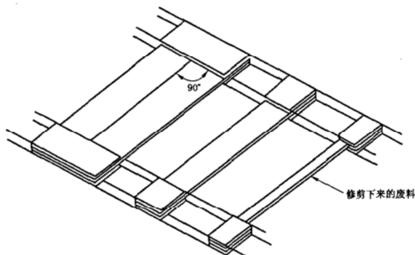
图 A.1 制备试样
