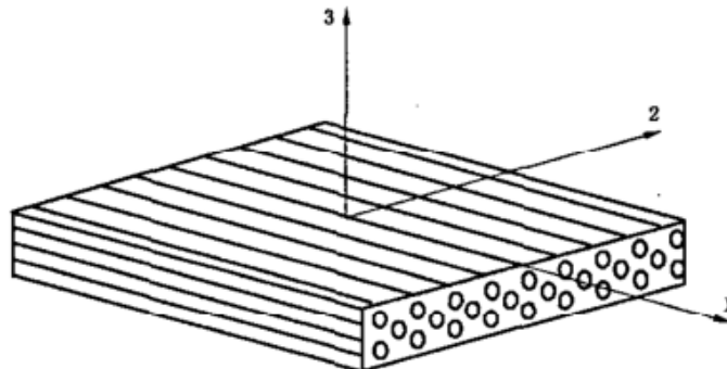
图 2 纤维增强复合材料的坐标轴
