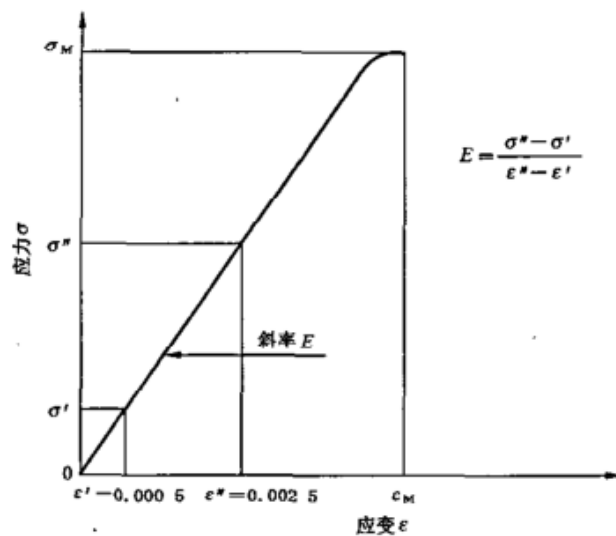
图 1 应力-应变曲线
